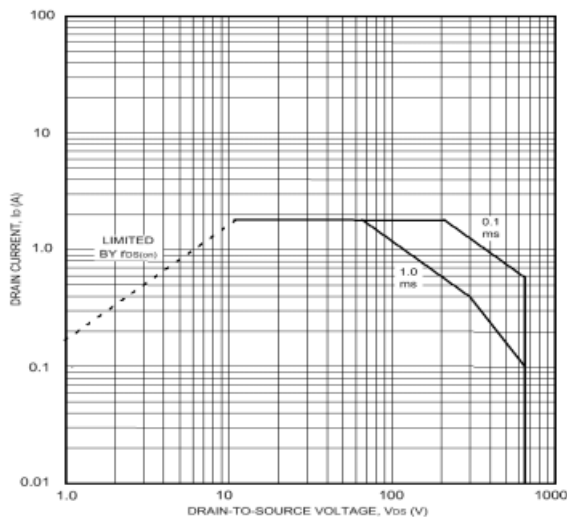
STR-A6159
